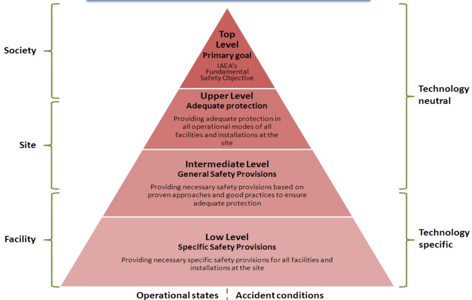
例：IAEAが提案する安全目標の階層構造
